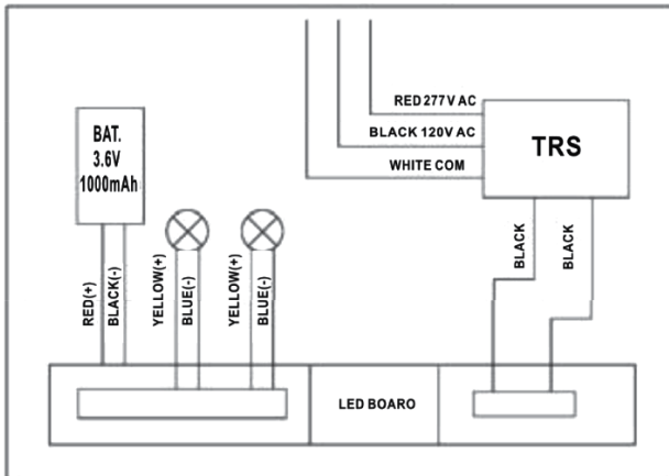
COMBO WIRING DIAGRAM:
